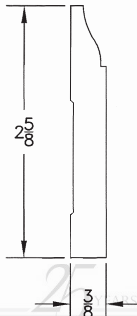
M-222 3/8 x 2 5/8
